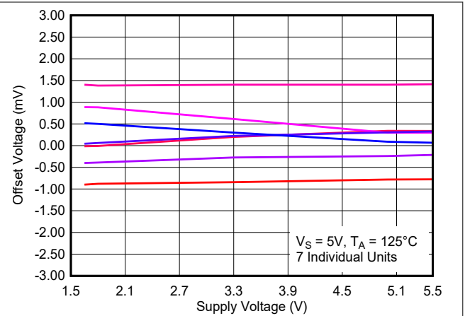
图 8-32. 失调电压与电源电压间的关系, 125°C
