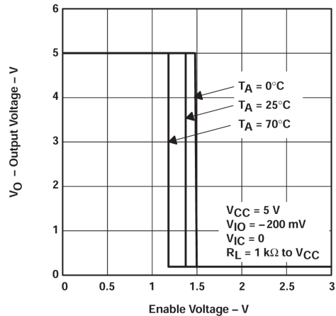
图 5-4. Output Voltage vs Enable Voltage
