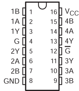
图 4-1. D 或 N 封装 (顶视图)
